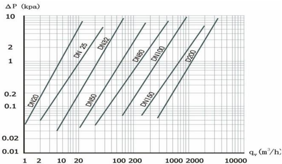
压力损失曲线
